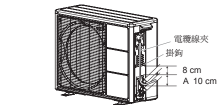
連接電纜的接線
