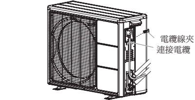
連接電纜的接線
